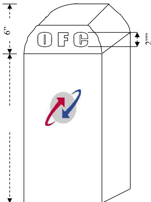
ELEVATION
